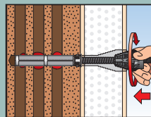
7 | Thermax eindrücken
