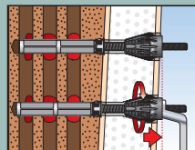
8 | Thermax bei Bedarf auf Abstand justieren
