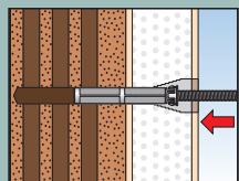
5 | Siebhülse einschieben
