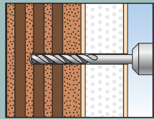
1 | Bohrloch herstellen
