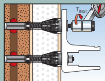
10 | Konsole befestigen
