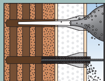
4 | Bohrloch reinigen
